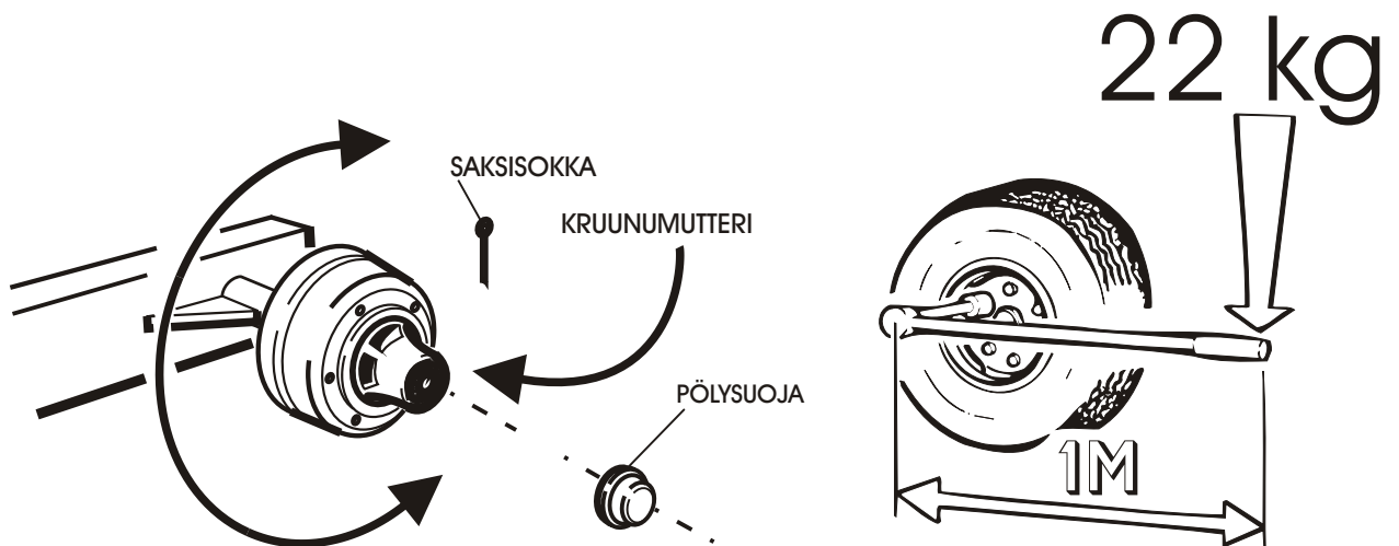
PYÖRÄNPULTTIEN KIRISTYS
