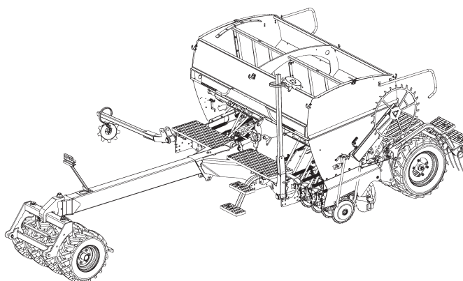
Kuva 10. Vetolaite ja aisa koottuna
