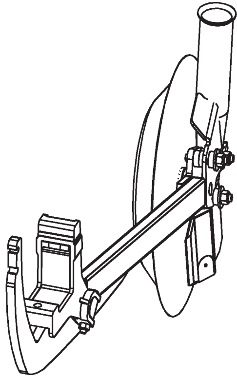
Kuva 102. S-mallin poskilevyn vaihto
