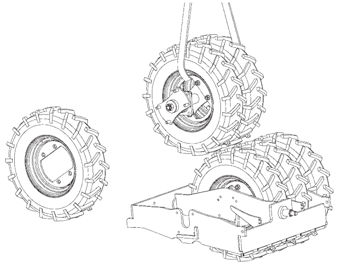
Kuva 100. Renkaan irrotus
