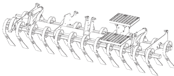
Kuva 92. Kaksirivinen etulata
