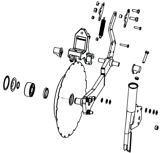
Kuva 104. M-mallin vantaan osat
