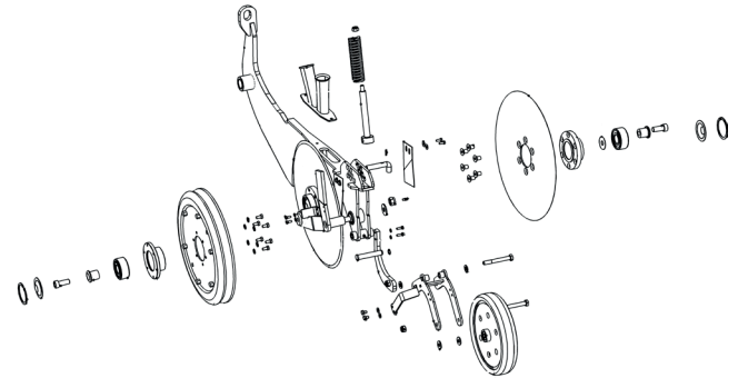
Kuva 107. D-mallin vantaan osat
