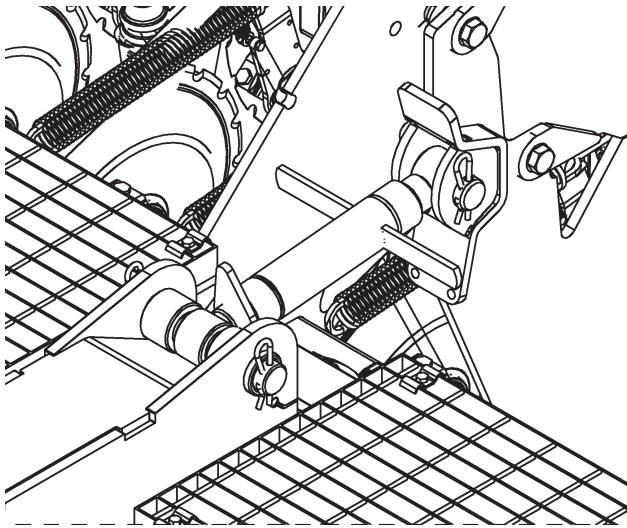
Kuva 30. Työntövarsi M- ja D-mallissa
