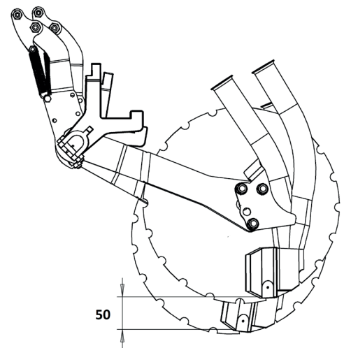
Kuva 44. Vannas lepo- ja työasennossa
