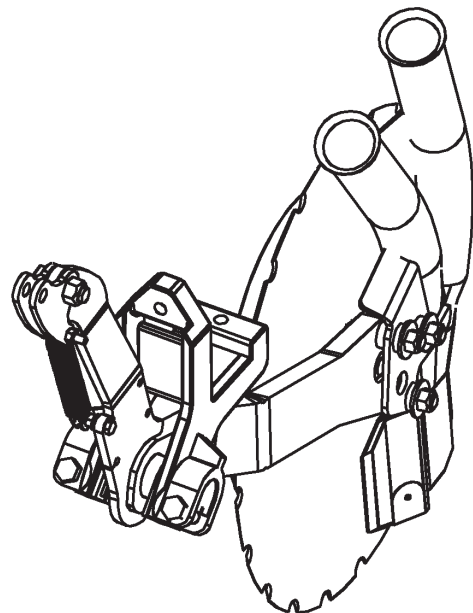
Kuva 105. M-mallin poskilevyn vaihto
