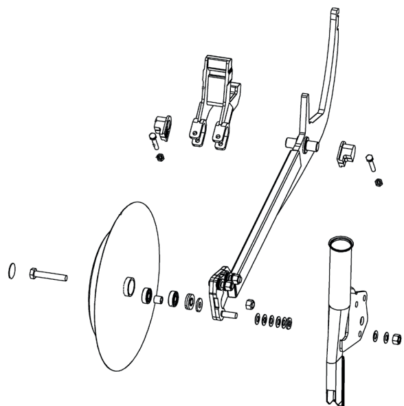
Kuva 101. S-mallin vantaan osat
